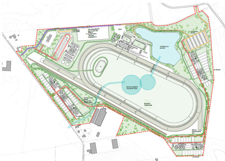
Figur 20. Reviderad situationsplan under våren 2025.
