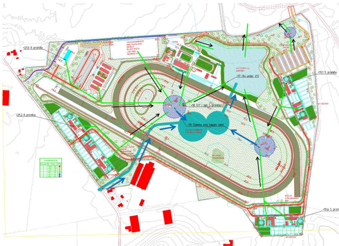
Figur 40. Föreslagen dagvattenhantering. Källa. Dagvattenutredning (WSP 2025).
