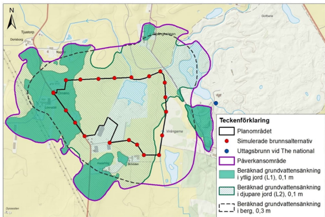
Figur 49. Simulerat påverkansområde för grundvattensänkning av ytligt grundvatten i jord (beräkningslager 1), djupare grundvatten i jord (beräkningslager 2) och grundvatten i berg. Källa. Hydrogeologisk utredning, WSP 2025.
